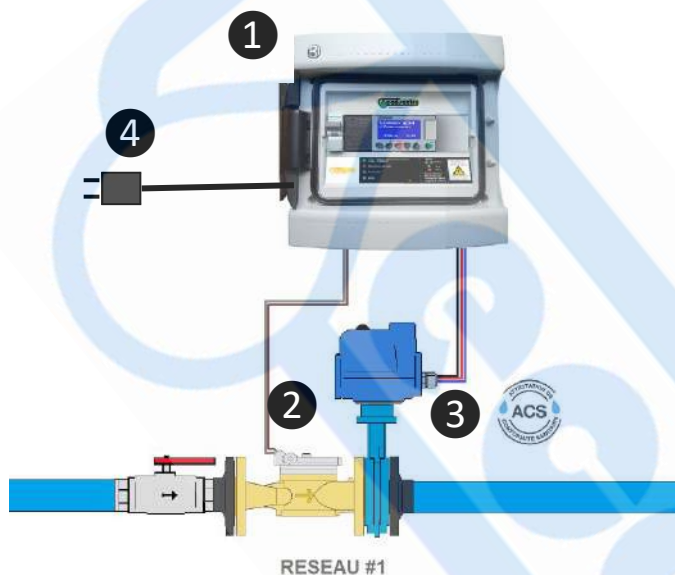
COFFRET M3 - 1 RESEAU D'EAU
